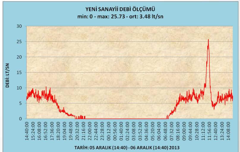
ÖRNEK DEBİ GRAFİĞİ
